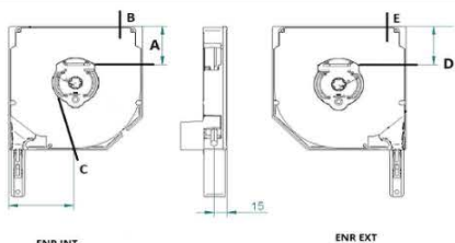
Sortie de manivelle et câble
