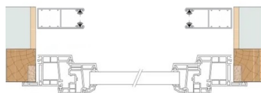
DISPO 1 Enroulement intérieur Pose en tableau
