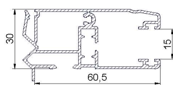
Coulisse ALU 60x30
