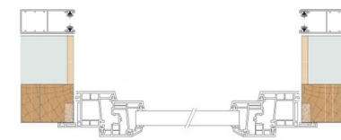
DISPO 3 Enroulement extérieur Pose en face
