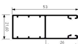
Coulisse alu 53x22
