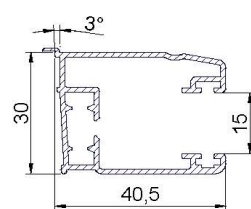
Coulisse ALU 40x30
