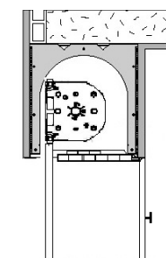
DISPO 5B - Coffre linteau
