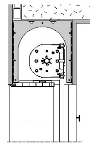
DISPO 5A - Coffre linteau
