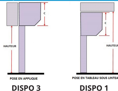
Disposition et sortie de caisson
