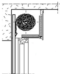
DISPO 1 Enroulement intérieur
