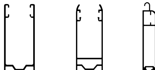
Coulisse alu 40x22 Coulisse alu 45x22 Lame finale alu 9mm
