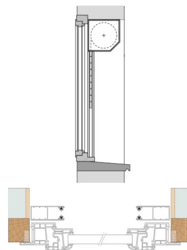
DISPO 2 Enroulement extérieur Pose en tableau
