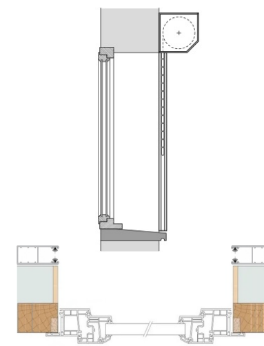
DISPO 3 Enroulement extérieur Pose en face
