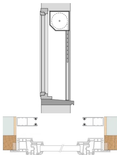
DISPO 1 Enroulement intérieur Pose en tableau
