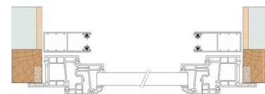
DISPO 2 Enroulement extérieur Pose en tableau
