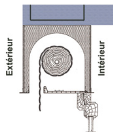
DISPO 5B - Coffre linteau Enroulement intérieur
