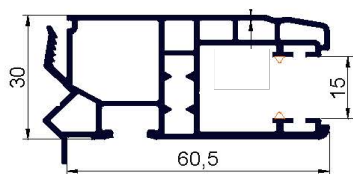
Coulisse reno PVC 60x30
