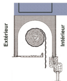
DISPO 5A - Coffre linteau Enroulement extérieur
